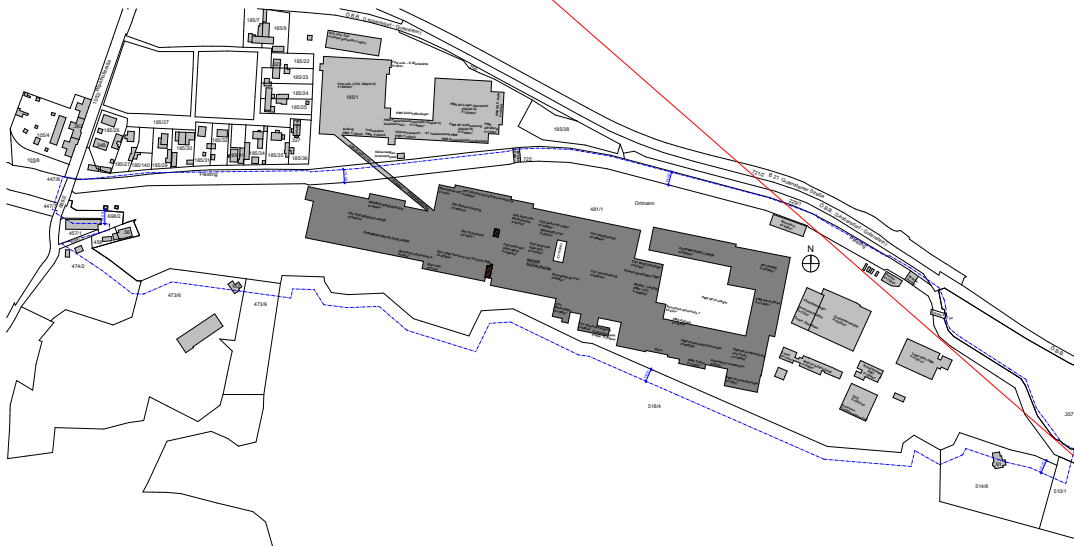
LAGEPLAN M 1:2000
