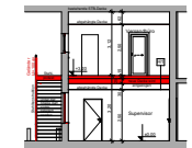
Schnitt A-A 1:100
