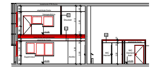
Schnitt B-B 1:100
